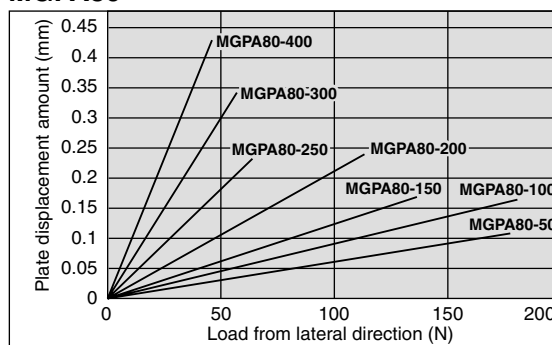
MGPA80
