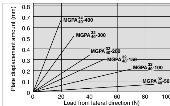
MGPA32/40
