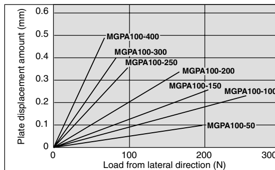
MGPA100
