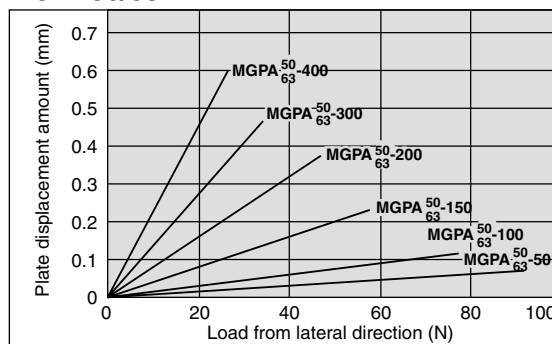
MGPA50/63
