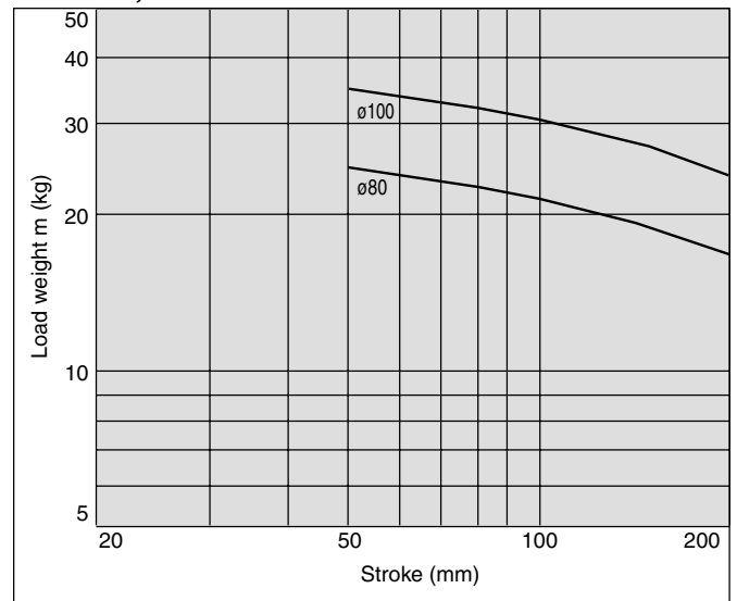
MGPL80, 100
